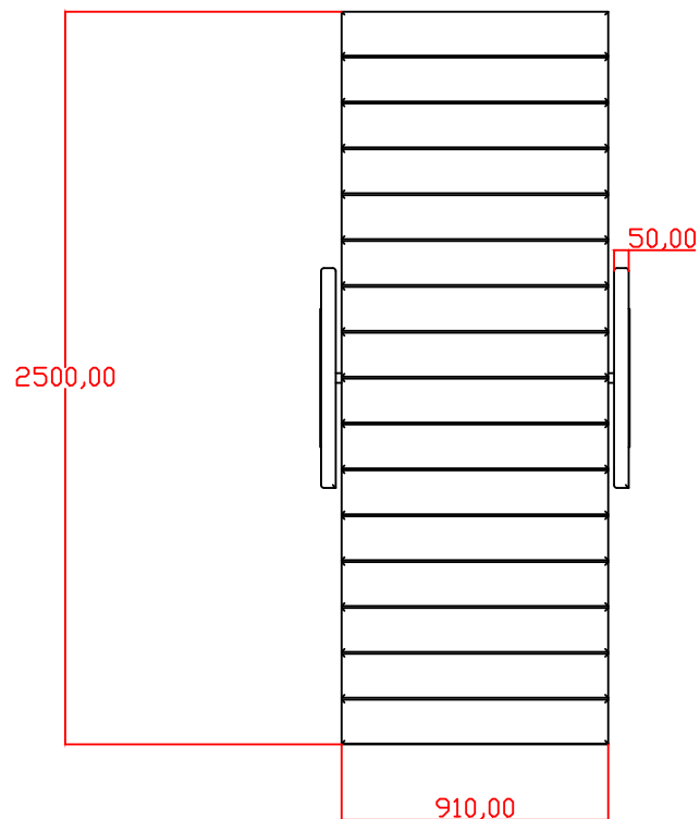
PLANTA BAIXA
