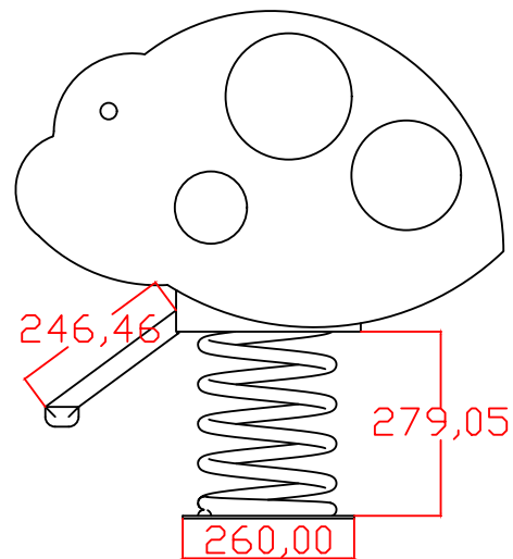
Vista Lateral
