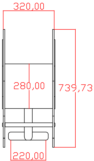
Vista Superior
