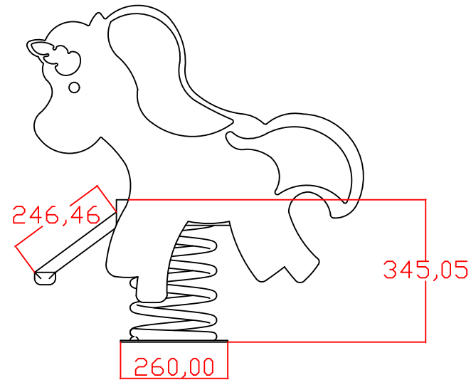
Vista Lateral
