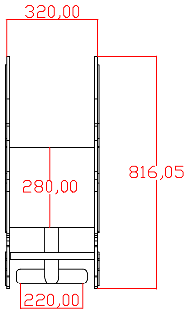
Vista Superior
