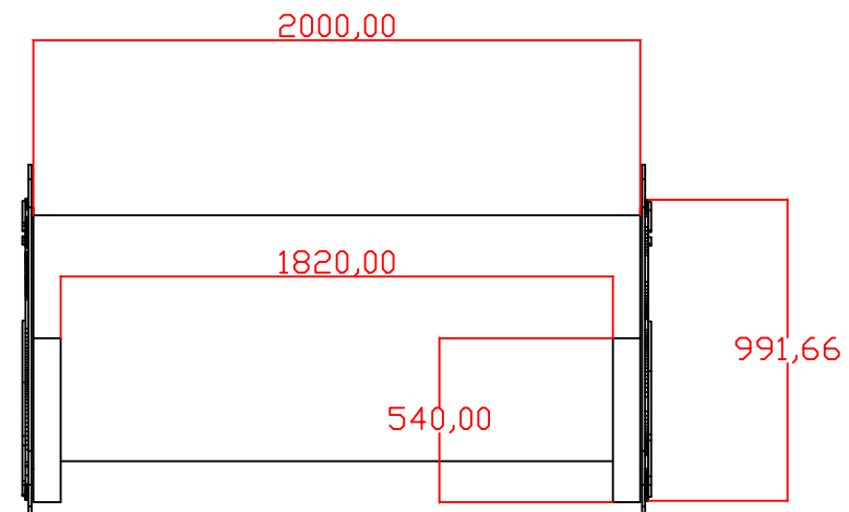
VISTA LATERAL
