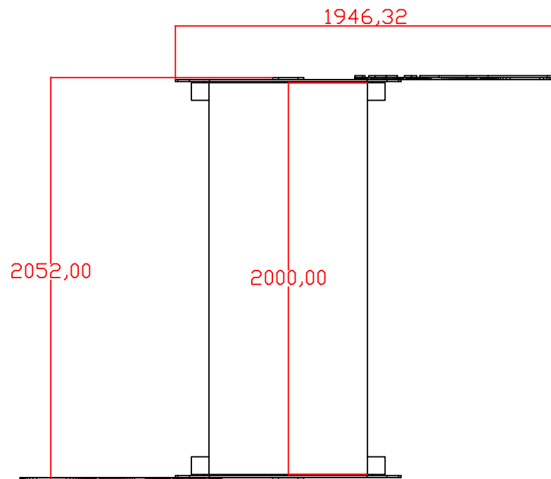
PLANTA BAIXA
