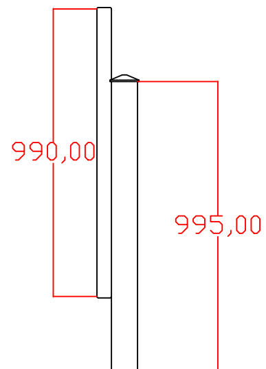
VISTA LATERAL
